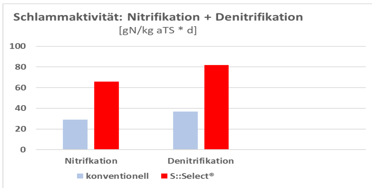
Bild: Höhere Schlammaktivität S::Select® gegenüber konventionell
