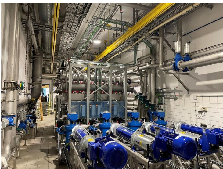
S::Select®-Anlage KA Damhusaen (350.000 EW), installiert in einer Maschinenhalle
